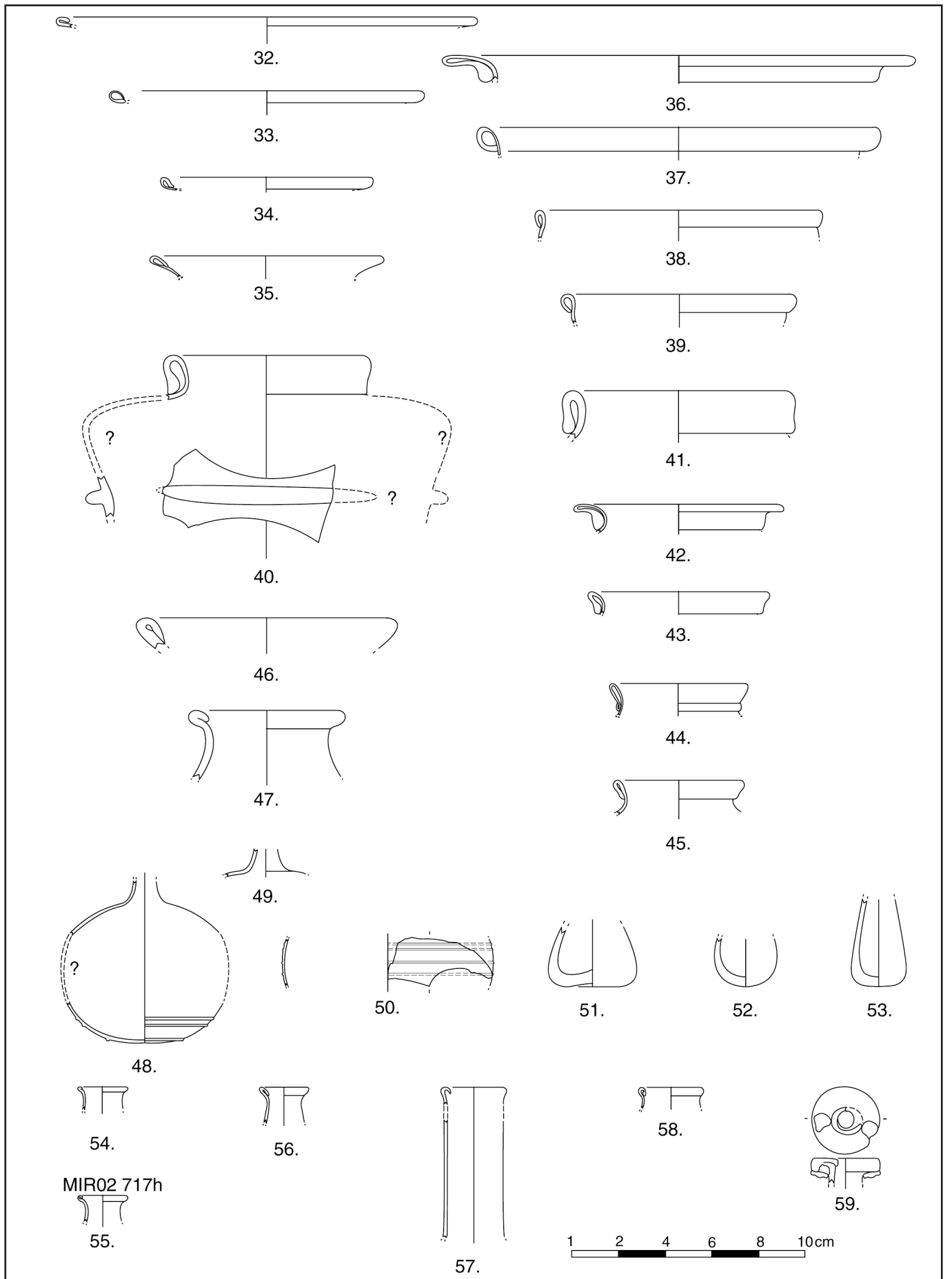
Pl.. 2.- Mobilier en verre de Mirebeau-sur-Bèze (verres à lèvre ourlée et petits flacons).
