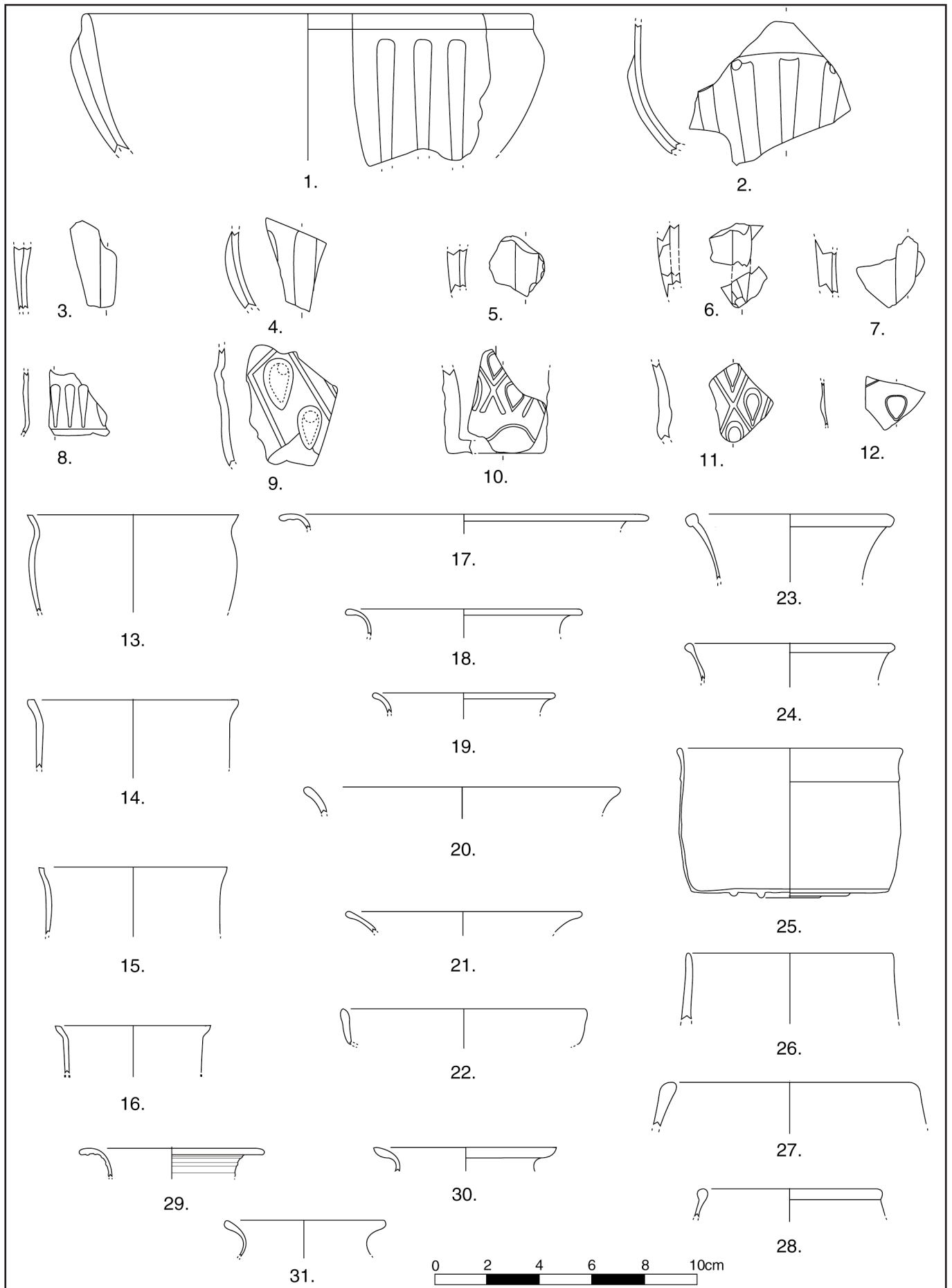
Pl. 1.- Mobilier en verre de Mirebeau-sur-Bèze (formes ouvertes).
